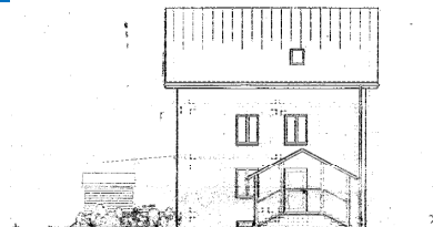
Ostfassade
