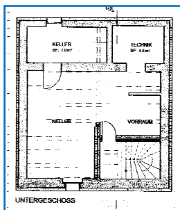
Untergeschoss
